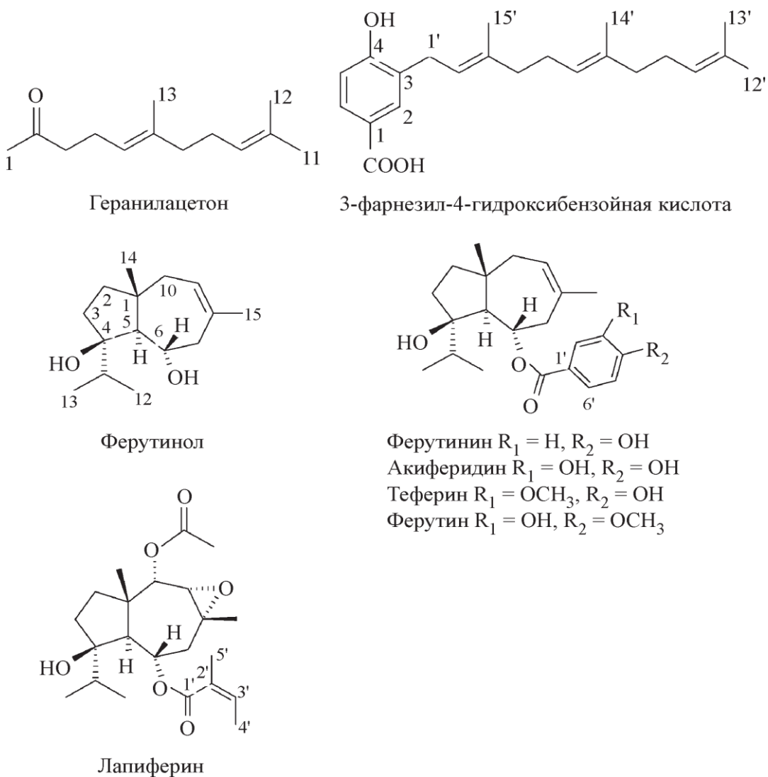
Сурет 1 - Ferula songarica өсімдігінің тамырынан алынған спиртті экстракттан бөлініп алынған қосылыстар.
