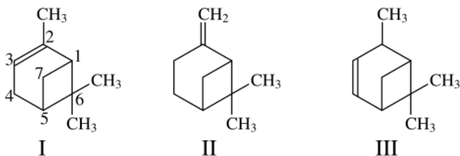
Сурет 2 - \alpha -пинен (I), \beta -пинен (II) және \delta -пинен (III) құрылымдық формулалары
